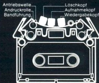
Prinzipdarstellung: Riemenantrieb
