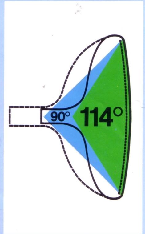
Konventionelle Röhre
