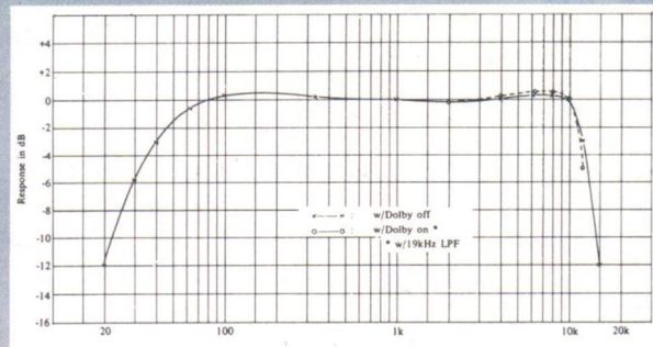
TC-161 SD Band Pegel Frequenzgang Über-Alles Normal-Band 30 dB unter Null VU
