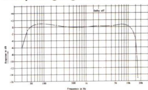
TC-134 SD Frequenzgang Über-Alles Band SONY C 60 CR Pegel 30 dB unter Null VU TC-134 SD Frequenzgang Über-Alles Band Normal-Band Pegel 30 dB unter Null VU
