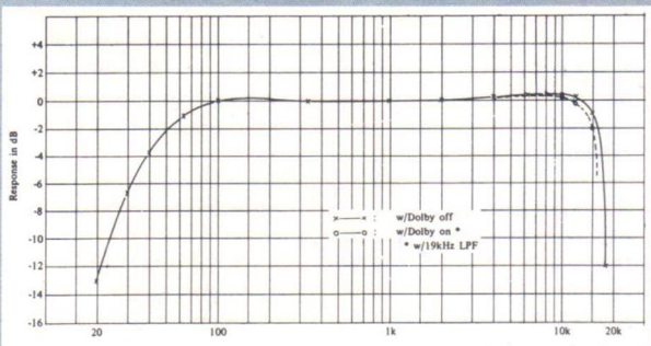
TC-161 SD Band Pegel Frequenzgang Über-Alles SONY C 60 CR 30 dB unter Null VU
