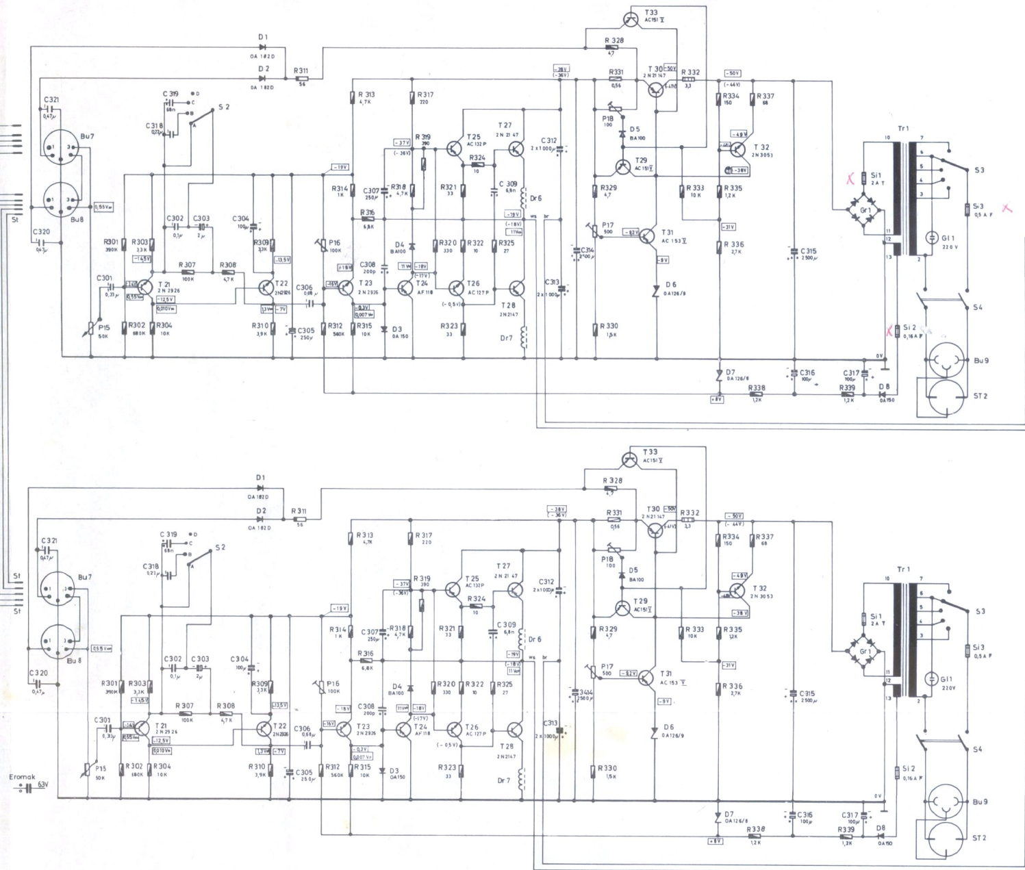
2 Leistungstrahler VKL 303
