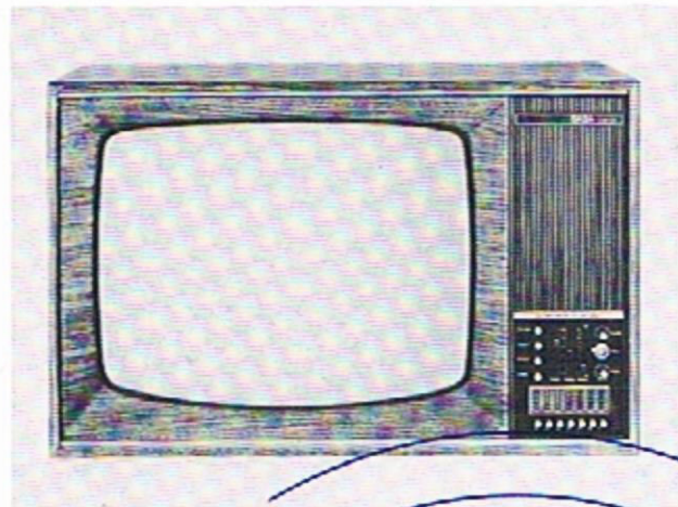
SABA Schaulnsland T 2500 color Phantastische Bildhelligkeit, leuchtende Farben. Vollelektronische Senderwahl. 7 Stationstasten. Vollautomatische Scharfabstimmung. Einfache Bedienung. Maße: 75,5 x 49,5 x 55,5 cm Festpreis (Grundausrüstung) DM 2298,-
