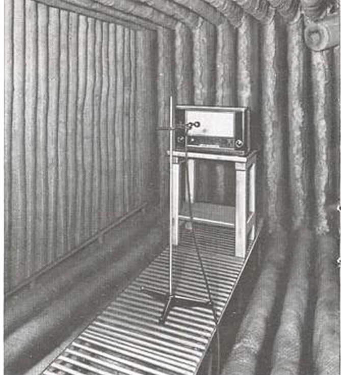
Schalltoter Meßraum
