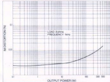
IM DISTORTION vs OUTPUT POWER
