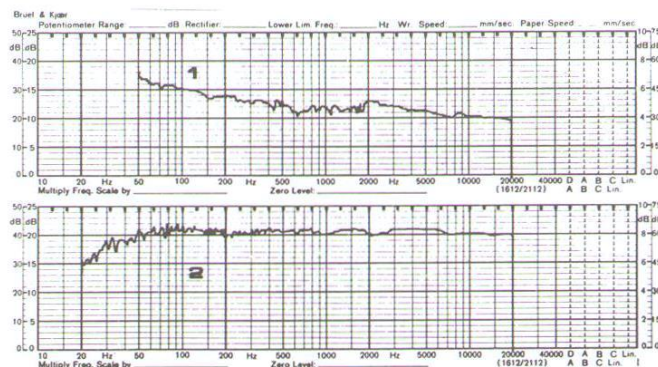
1. Phasenverlauf 2. Amplitudenverlauf des Leistungsschaltwandlers DEFENDER
