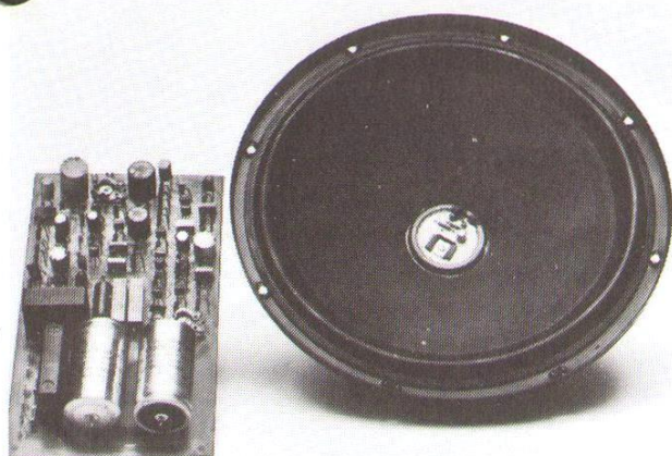
Lautsprecher mit eingebautem Sensor und dazugehörige Elektronik
