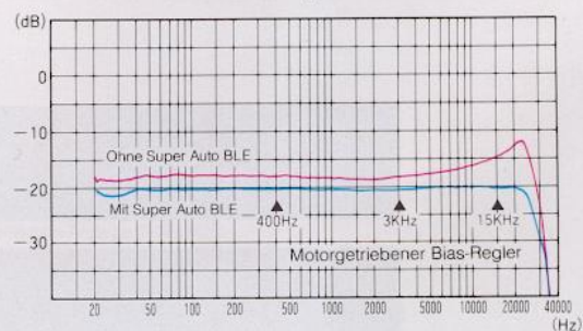
Aufnahme/Wiedergabe-Frequenzgang ohne und mit Super Auto BLE
