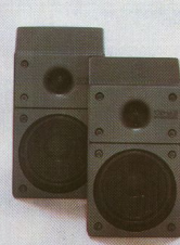
CS-X3 Miniatur-2-Wege-2-Lautsprecher-Box nach dem Prinzip der geschlossenen Schallwand und mit luftgedämpfter Aufhängung in gegossenem Alu-Gehäuse. 10-cm-Konus-Lautsprecher, 2,5-cm-Kalotten-Hochtöner in getrennten Gehäusen. Für Regalaufstellung oder Wandaufhängung. Impedanz 6,3 Ohm. Frequenzbereich 50–20 000 Hz. Maximale Belastbarkeit 50 Watt. Abmessungen (Hx B x T): 188 x 118 x 112 mm.
