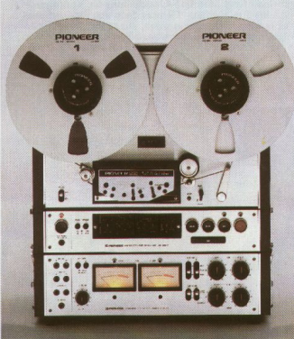
RT-2022 riemengetriebene Spulentonbandmaschine mit Studio-Geschwindigkeit 3-Motoren-3-Kopf-System, gebaut nach professionellen Spezifikationen mit Bandgeschwindigkeiten 19 und 38 cm/s. Separate Einheiten für Bandtransport, Verstärker und Kopftträgerplatte. Fortgeschrittene Tonbandfreunde können durch einfaches Austauschen der Kopftträgerplatte von 2-Spur-2-Kanal auf 4-Spur-4-Kanal und durch Zusatz eines weiteren Verstärkers TAU-11 bestmögliche Flexibilität und Einsatzmöglichkeiten erreichen. Enthält sowohl NAB- als auch IEC-Entzerrung, stufenlos einstellbare Vormagnetisierung, eingebauter Testoszillator. Tonhöhenchwankung \pm 0,06\% nach DIN, Spulengröße 26,5 cm.
