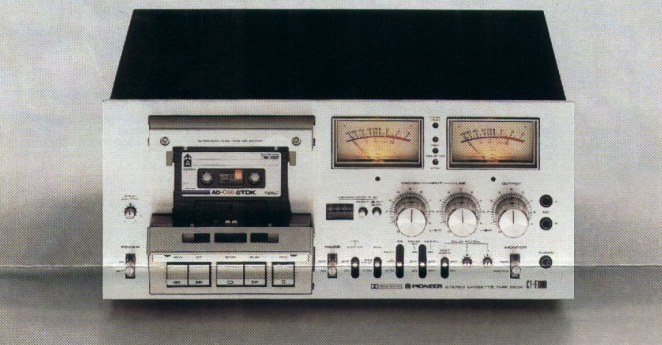
CT-F 1000 2 Motoren-3-Kopf-Dolby-Cassettenmaschine Das Gerät mit allem: automatische Chromumschaltung, Anzeigeleuchtung, Mehrfach-Umschaltung für Vormagnetisierung und Entzerrung, Geschwindigkeitsfeinregulierung, Mikrofon/Line-Einmischung, Memory-Stop und Play, automatische Fangvorrichtung für Bandschlaufen, vollautomatischer Stop, magnetgesteuerter Antrieb, direkt umschaltbar, und eingebauter Testoszillator. 3-Kopf-Aufbau mit Aufnahme/Wiedergabekopf aus Einkristall-Ferrit erlaubt direkte Hinterbandkontrolle. Tonhöhen-schwankung \pm 0,15\% nach DIN, Frequenzgang 30–17.000 Hz \pm 3 dB bei Fe/Cr-Band.
