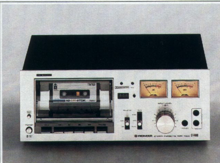
CT-F 4040 Dolby-Cassettenmaschine mit vollautomatischem Stop Mit den von Pioneer entwickelten Cassettenhalterungen, die ohne die sonst üblichen Auswurfmechanismen auskommen. Beleuchtetes Cassettenfach mit spezieller Markierung zur Anzeige des Bandvorrates. Elektronische Stummschaltung zur Unterdrückung aller Schaltergeräusche und Aufnahme/Wiedergabekopf aus Hart-Permalloy, Löschkopf aus Ferrit. Tonhöhen-schwankung \pm 0,18\% nach DIN, Frequenzgang bei Chromband 40–15.000 Hz \pm 3 dB.
