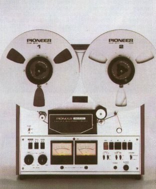
RT-1011 L 4-Spur-riemengetriebene Spulentonbandmaschine Drei Motoren, drei Köpfe, zwei Geschwindigkeiten 9,5 und 19 cm/s. Magnetgesteuert mit volllogischem Bandantrieb, eingerichtet für Schalltrübbetrieb und Wiedergabe. Hyperbolische Tonköpfe aus Permalloy, Hysteresis-Synchron-Motor zum Tonwellenantrieb und spezielle Induktionsmotoren für die Spulenantriebe. Eingerichtet für 26,5 cm, professionelle Spulen für besonders lange Spielzeiten. Vierfach-Umschaltung für Vormagnetisierung und Entzerrung und viele weitere Einzelheiten. Frequenzgang 30–24 000 Hz nach DIN bei 19 cm/s. Tonhöhenchwankung \pm 0,15\% nach DIN bei 19 cm/s.
