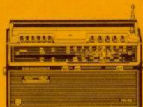
Radio Recorder de Luxe RR 622 UKW, MW, LW, 2 x KW (49-m-Band/13-41-m-Band), eingebautes Cassetten- Tonbandgerät, eingebautes Netzteil
