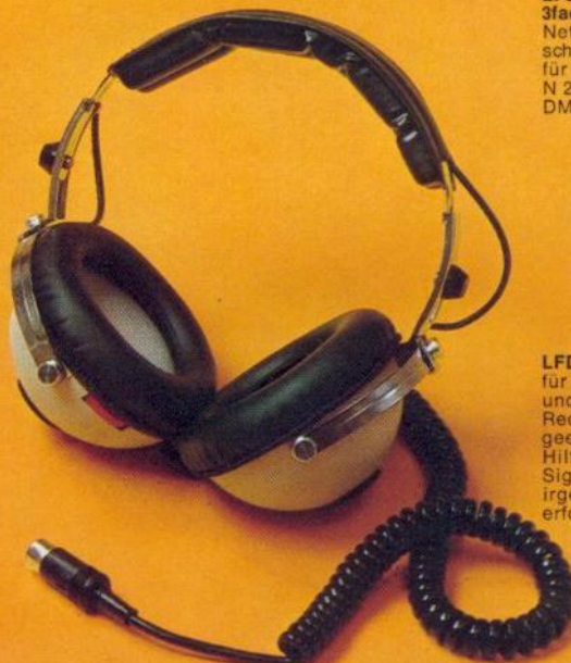
N 6302 HiFi-Stereo-Kopfhörer für N 4416, N 4418, N 4510, N 4450 sowie zum Anschluß an HiFi-Verstärker. Frequenzbereich: 16–20 000 Hz. Mit Regler zur Veränderung der Stereo-Breitenbasis. Gewicht 450 g. DM 175,—*
