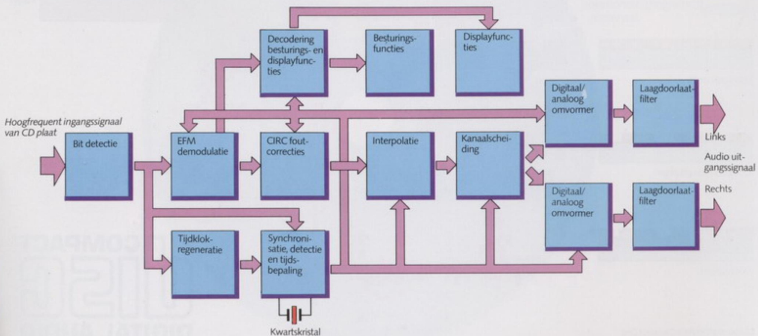
Het CD decodingscircuit hier afgebeeld tegen de achtergrond van een sterk vergroot LSI.
