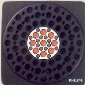
EN 8359 5"-Breitbandsystem Belastbarkeit 8 Watt Übertragungsbereich 100–12 500 Hz
