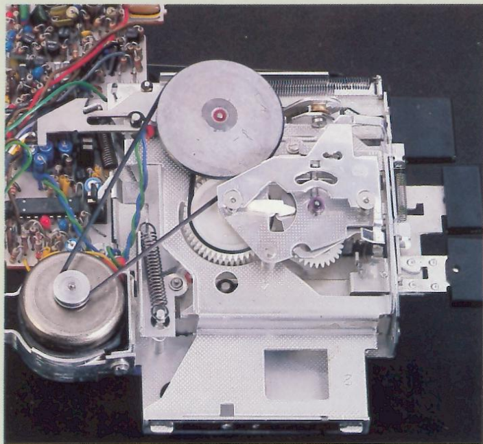
Philips-Cassettenlaufwerk
