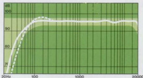
Perfect-rechte frequentiecarakteristiek van uiterst laag tot uiterst hoog.
