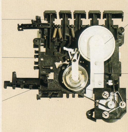
Makrolon für die Schwungmasse: extrem glatt und dennoch griffig für guten Lauf der Antriebspeise. (Cadmierte Stahlplatte erhöht die Masse.)
