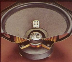
Das quadratische piezokeramische Element in der runden Printplatte ist das Herzstück des MFB-Lautsprechers.
