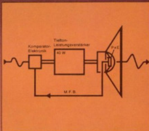
Schema des MFB-Systems mit PXE-Wandler, Komparator-Elektronik und Tiefen-Leistungsverstärker
