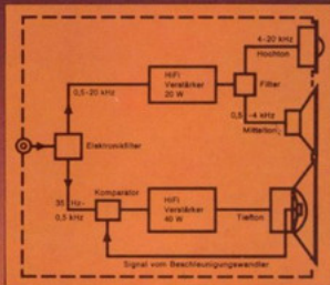
Die MFB-Box im schematischen Aufbau: 3-Weg-Box mit 2 integrierten Verstärkern für Mittel-/Hochton und Tiefen mit PXE-Wandler.
