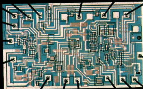
Ein integrierter Schaltkreis in vielfacher Vergrößerung.
