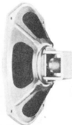
Universal-Lautsprecher (oval)
