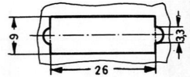
Chassisdurchbruch
