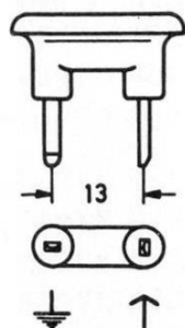
AM-Antennenstecker
