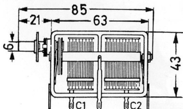
Zweifach-Drehkondensator
