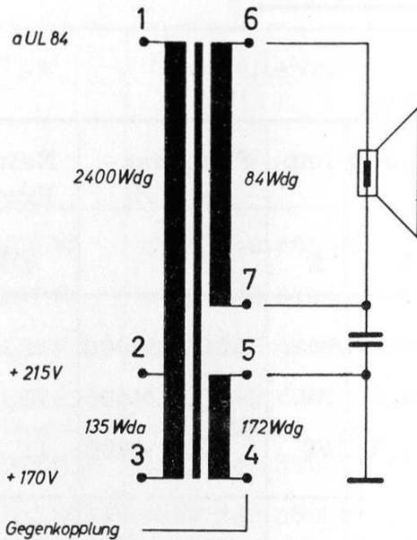
Schaltung
