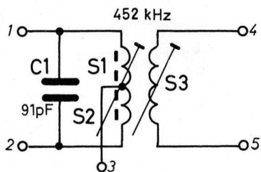
Schaltung
