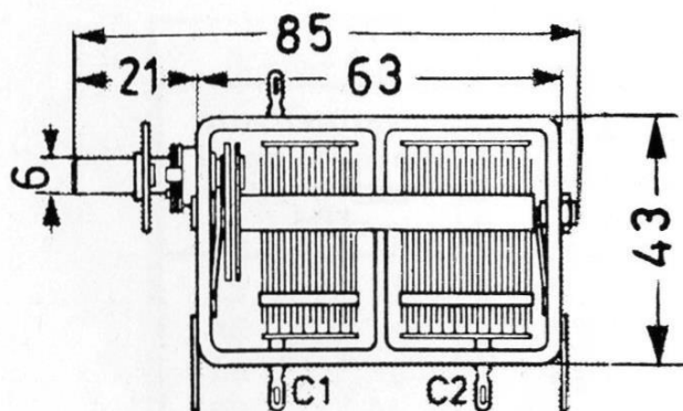
Zweifach-Drehkondensator
