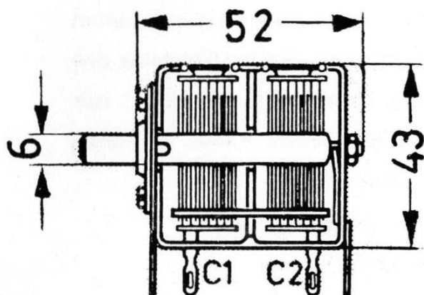
Zweifach-Drehkondensator
