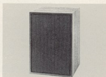
NG 1215 Lautsprecherbox für alle Geräte. Impedanz: 8 Ohm Belastbarkeit: 6 Watt Frequenzgang: 70 Hz — 18 kHz Edelholzgehäuse (s. Seite 13) DM 59,—*
