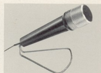
8302 Dynamisches Breitband-Mikrofon für alle Geräte. Richtcharakteristik: Niere Empfindlichkeit: 0,24 mV/ubar Impedanz: 500 Ohm Frequenzbereich: 80 Hz — 19 kHz Stativgewinde 3/8"
