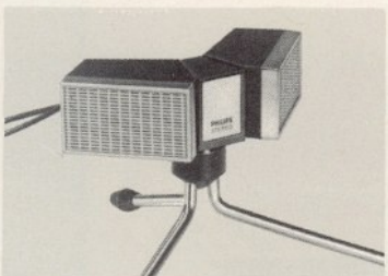
EL 1979 Dynamisches Stereomikrofon für 3312, RK 37 S, RK 57 S, 4408 mit 2 trennbaren Systemen Empfindlichkeit: 0,33 mV/ubar Impedanz: 500 Ohm (je Kanal) Stativgewinde 3/8"
