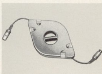
NG 1206 Verlängerungsleitung 6 m, mit Kabelhaspel. Verwendbar für alle Mono- und Stereo-Mikrofone mit 200 und 500 Ohm Impedanz. Mit 5-poligem Normstecker und 5-poliger Normbuchse. DM 23,—*
