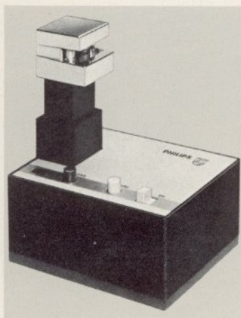
EL 1995 Dia-Steuergerät zur Steuerung automatischer Projektoren. Für alle Tonbandgeräte. Impulslage auf Spur 4. Impulsfrequenz: ca. 1000 Hz. Transistorisiert. Batteriebetrieb (mehr als 100 Std. Betriebsdauer). Drucktastensteuerung. Löschanzeige. Impulslöschung. Höhenverstellung. DM 125,—*
