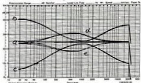
3 Regelumfang der Klangregler bei maximaler Anhebung bzw. Absenkung
