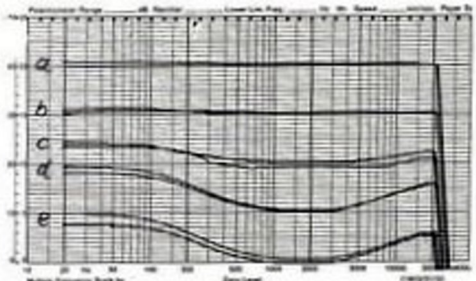
4 Frequenzgang bei gehöriger Lautstärkeregelung gemessen bei 6 dB unter Vollaussteuerung für die Reglerstellungen: a) 0 dB b) -10 dB c) -20 dB d) -30 dB e) -40 dB
