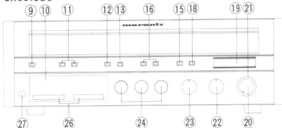
Figure 7. Front Panel Figure 7. Face avant Abbildung 7. Gerätevorderseite
