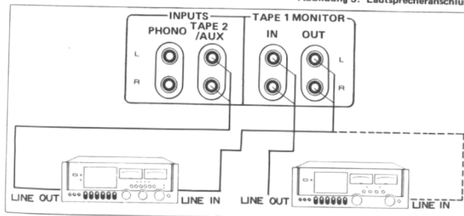
Figure 6. Raccordement typique de deux magnétophones Abbildung 6. Beispiel für den Anschluß zweier Bandgeräte
