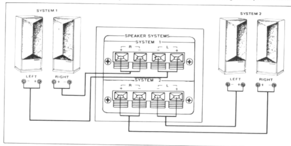
Figure 5. Raccordement des haut-parleurs Abbildung 5. Lautsprecheranschluß
