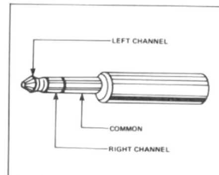
Figure 4. Stereophone Plug Figure 4. Fiche pour écouteurs Abbildung 4. Kopfhörerstecker
