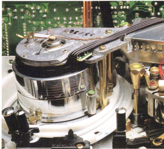
Schrägschurvideokopf
