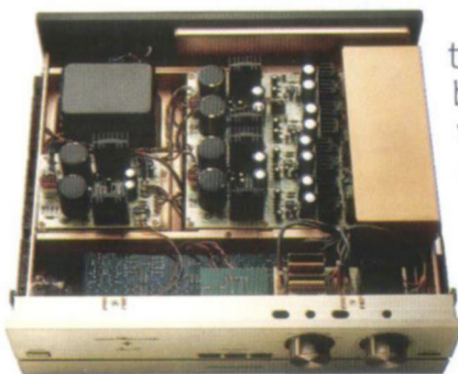
Innenansicht des Vorverstärkers SC-11.
