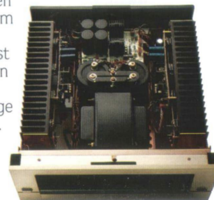
Innenansicht des Endverstärkers SM-11.
