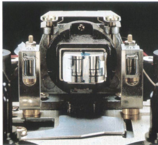
Schwenkkopf-Mechanismus mit Tonköpfen aus Super Hard Metal Alloy.
