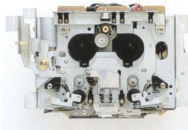
Hochwertiges Laufwerk aus Metall beim Cassettendeck.
