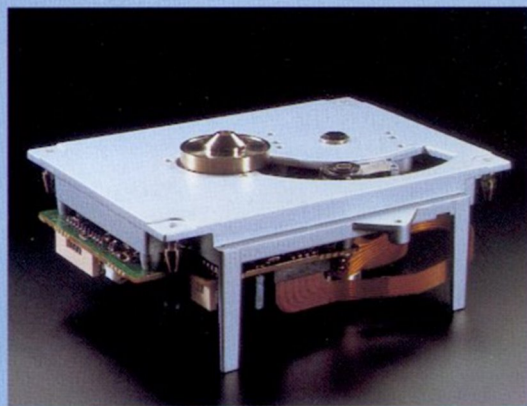
Laser-Ablese-Einheit
