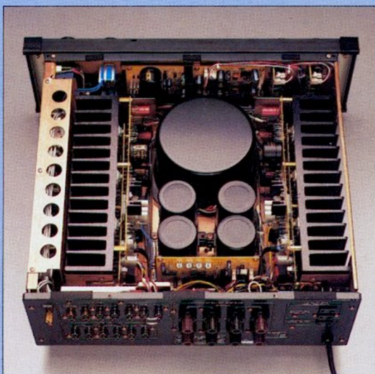
PM-94 Innenansicht
