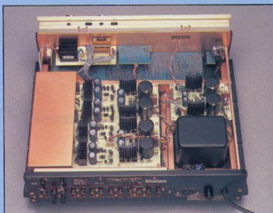
SC-11 Innenansicht
