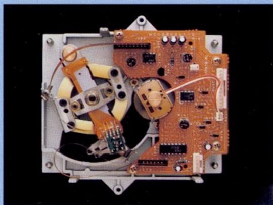
Laser-Ablese-Einheit (Rückansicht)
