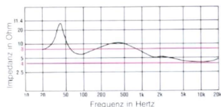
Impedanzkurve für typisches 30-cm/3-Weg-Lautsprecher-system, angegeben mit 8 Ohm.
