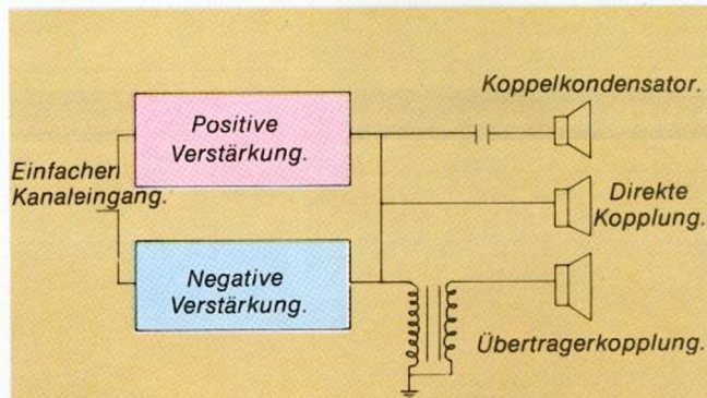
Verschiedene Arten der Kopplung von Ausgangsschaltungen.
