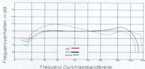
Frequenz Durchlassbandbreite
