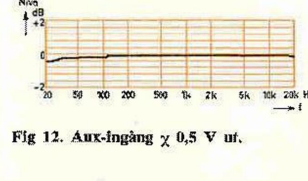
Fig 12. Aux-ingång x 0,5 V ut.
