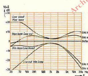
Fig 9. Aux Input: Kombinationen av tonkontroller och filter. Läge 400 Hz resp 2 kHz. Beteckningarna = kontrollernas mark.
