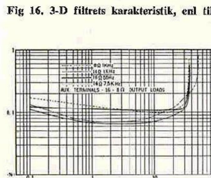
Fig 16. 3-D filterns karakteristik, en tillv.
