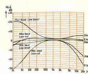
Fig 10. Samma som i fig 9, men med kontrollerna i läge 200 Hz–4 kHz.
