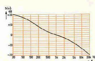
Fig 6. Frekvenskurva gällande förförstärkardelen. ≈ 0,5 V ut. (Phono 1).
