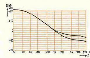
Fig 11. Karakteristiken för Tape Head.
