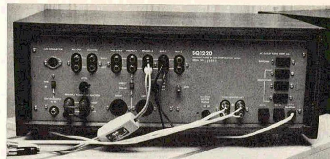
Fig 4. Bakre panelen på förstärkaren. Längst med tv utgången för »3 D-kanal» och över den omkopplaren till de, bredvid anslutningarna som förenar/avskiljer förstärkaren från effekt delen. Över de två uttagen för extra transformatorer syns omkopplaren för dessa. På vänstersidan finns också nivåreglaget för slutsteget. På höger sida sitter ner till, bredvid högtalarnanslutningarna, omkopplaren för dämpfaktörval. Nätledens reglage längst th. (Foto RT)
