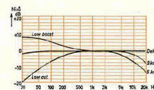
Fig 7. Aux Input: Hög- och lågpassfilterns karakteristik. Beteckningarna = kontrollernas mark.
