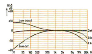
Fig 7. Aux Input: Hög- och lågpassfilterns karakteristika. Beteckningarna = kontrollernas mark.
