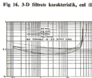
Fig 16. 3-D filterns karakteristika, en tillv.
