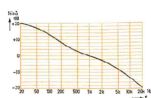
Fig 6. Frekvenskurva gällande förförstärkardelen. \approx 0,5 V ut. (Phono 1).
