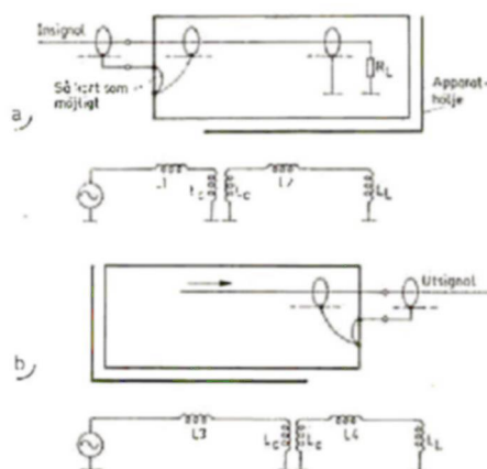
Fig 3 a—b. Anslutning av skärm till chassiskontakt vid (a) ingång på frontpanelen, (b) utgång på bakpanelen.
