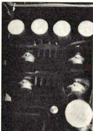
Fig 18, a och b: Två inblickar i förstärkaren med dess kretskortutbyggnad. Märk de stora kyl-elementen!
