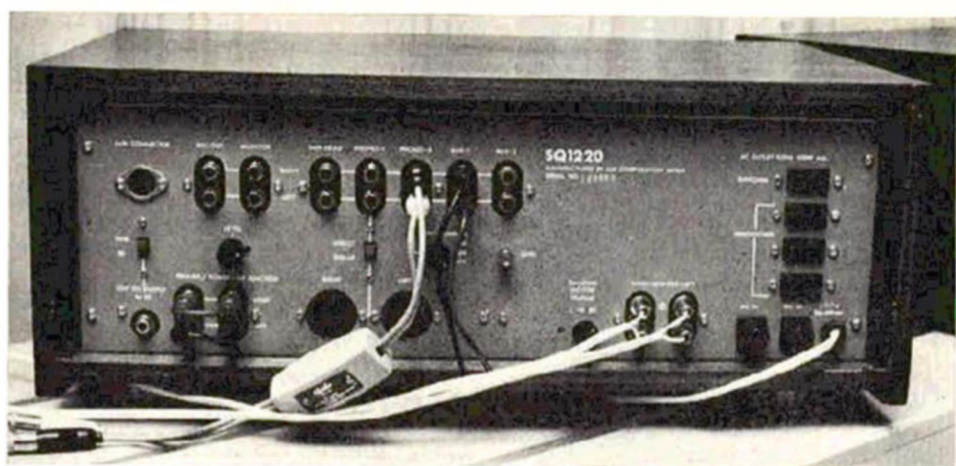
Fig 4. Bakre panelen på förstärkaren. Längst ned i v utgången för »3 D-kanalen» och över den omkopplaren till do, bredvid anslutningarna som förenar/avskiljer förförstärkaren från effektdelen. Över de två urtagen för extra transformatorer syns omkopplaren för dessa. På vänstersidan finns också nivåreglaget för slutsteget. På höger sida sitter närtill, bredvid högtalranslutningarna, omkopplaren för dämpfaktorval. Nätdelens reglage längst th.
