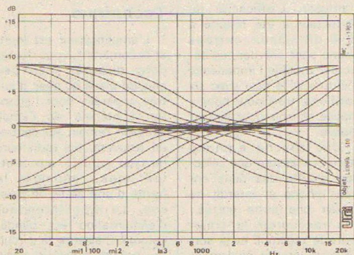
Courbe A. - Courbes de correction de timbre et réponse des filtres passe-haut et passe-bas.
