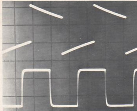
5 Das Rechteckübertragungsverhalten über alles (CL 350 + M 150)
