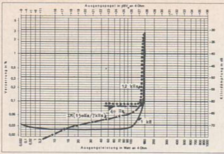
2 Das Leistung-Verzerrungs-Diagramm
