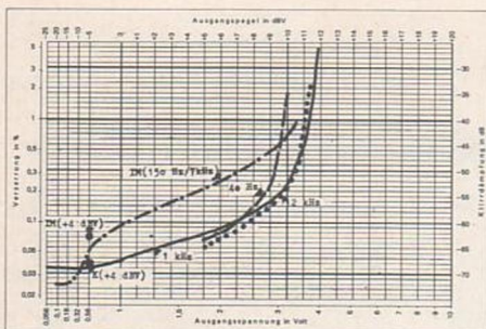
2 Das Leistungs-Verzerrungs-Diagramm
