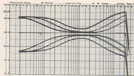
5 Klangreglerkurven mit den Einsatzfrequenzen 150, 300 und 600 Hz im Baß, 1,5, 3 und 6 kHz in den Höhen, gemessen in beiden Kanälen. Die lineare Kurve ergibt sich in Stellung „defeat“ der Klangregler und Filter
