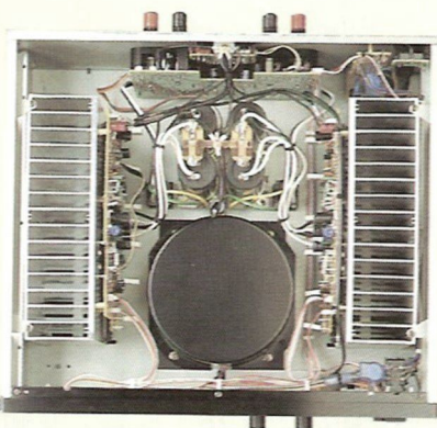
Symmetrischer Aufbau
