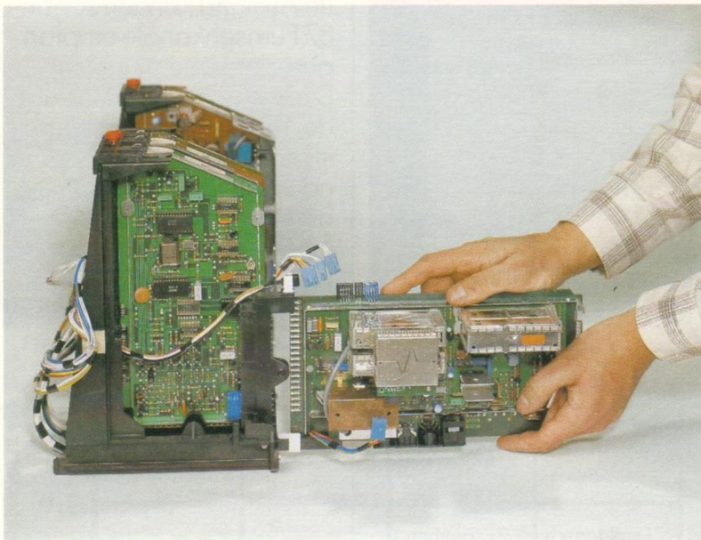
Im Servicefall ist das steckbare Modul rasch und problemlos ausgewechselt.
