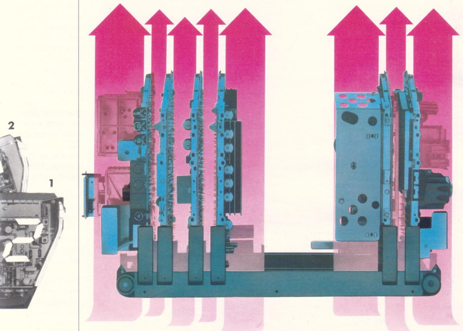
Die senkrechte Anordnung der Moduln ermöglicht eine kaminartige Luftzirkulation mit äußerst günstiger Kühlwirkung.
