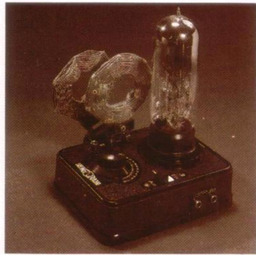
1926: Die von LOEWE OPTA entwickelte „Dreifach-Röhre“ mit integrierter Schaltung macht erstmals betriebs-sichere Radios möglich.
