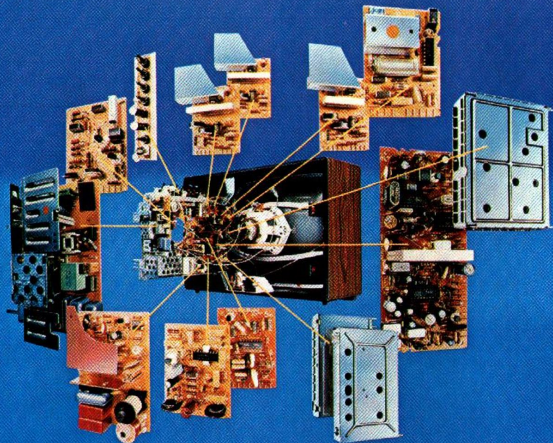
Modul-Chassis C 5000 Das Modul-Chassis C 5000 mit 14 steckbaren Funktionsmodulen. Das bedeutet: Das Erkennen und die Beseitigung von Störungen ist einfacher geworden.
