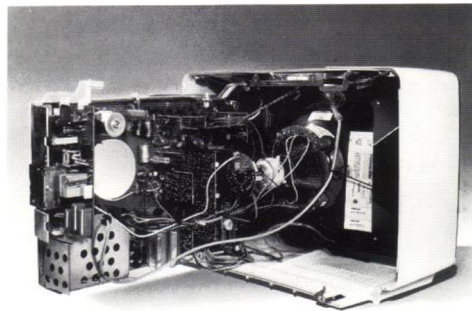
Servicefreundlicher Aufbau mit 8 Modulen, unverwechselbaren Steckverbindungen, Quick-Service-System in Verbindung mit einem Diagnose-Adapter, kennzeichnen beim Loewe CP 42 Color sensotronic die fortschrittliche Technik der Loewe-Fernsehgeräte.
