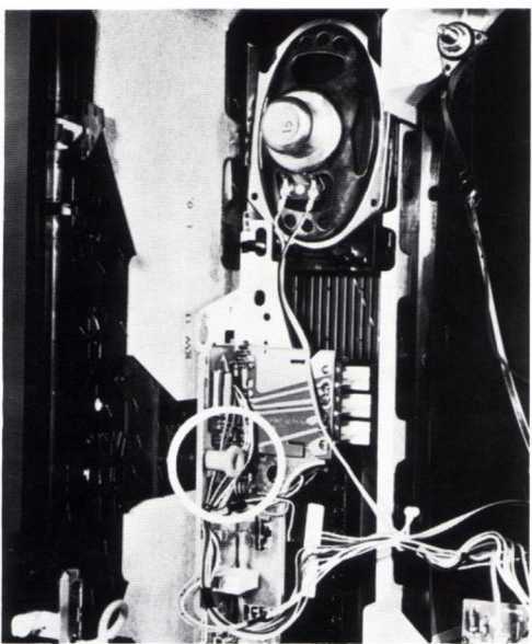
Haupt-Chassis in seiner Halterung nach hinten herausgezogen
