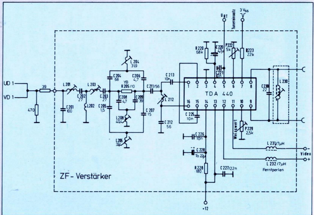
Gesamtschaltung des Bild-Zwischenfrequenz-Verstärker Modul
