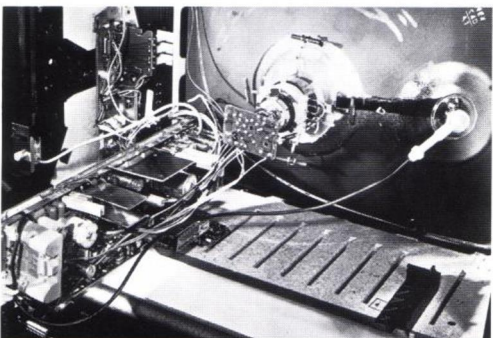
Haupt-Chassis um 90° abgewinkelt eingesteckt, so daß beide Seiten der Platine leicht zugänglich sind. Die Kabelverbindungen sind so lang bemessen, daß das Chassis in allen Servicestellungen voll betriebsfähig bleibt.
