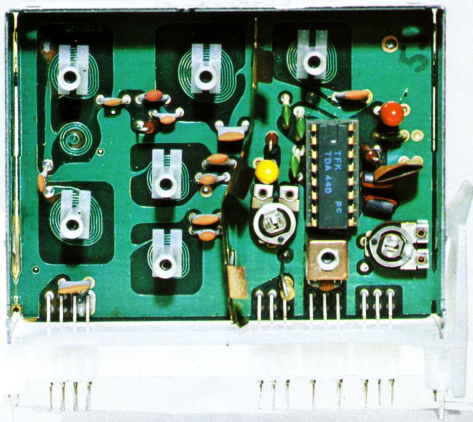
Ansicht des geöffneten ZF-Bausteins mit Fassung
