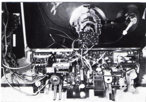
Haupt-Chassis senkrecht in die Halterung eingesteckt
