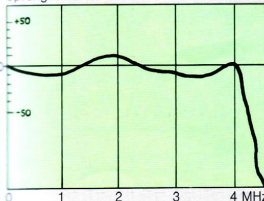
Gruppenlaufzeitkurve (gemessen mit Vorentzerrung über EE68F)
