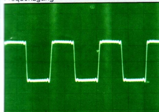
Sprungverhalten — 250 KHz Rechteck
