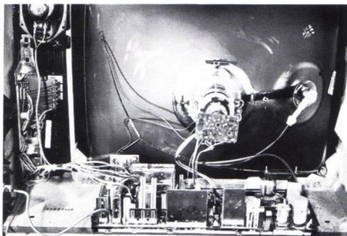
Haupt-Chassis in Betriebsstellung
