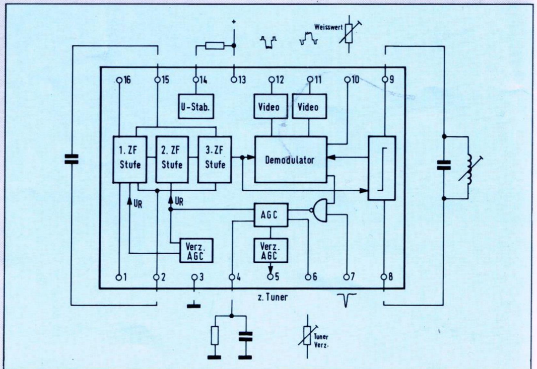
Blockschaltbild des integrierten Schaltkreises TDA 440 für den Bild-Zwischenfrequenz-Verstärker Modul
