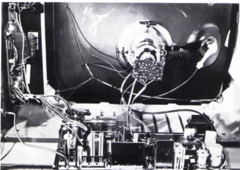
Haupt-Chassis in seiner Halterung nach hinten herausgezogen
