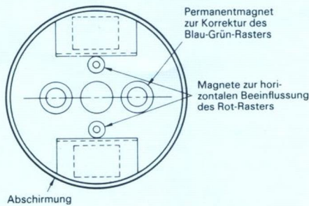
Die Austrittsöffnungen an der Stirnseite des Elektronensystems enthalten kleine Magnete zur Rasterkorrektur.
