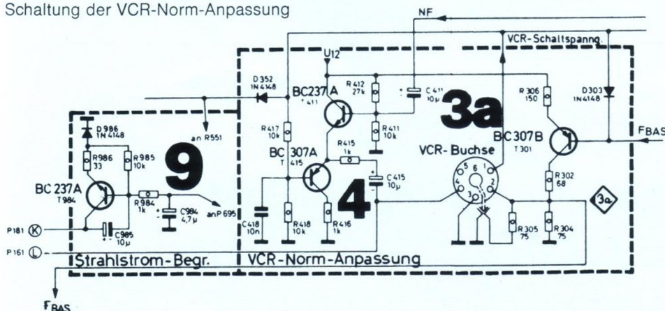
Schaltung der VCR-Norm-Anpassung
