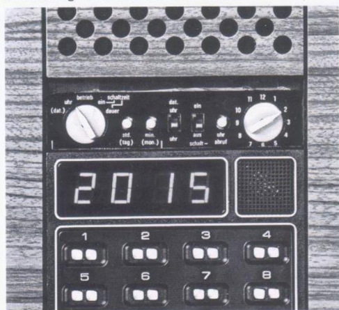
Stellfeld des Loewe CT 4070 für Uhrzeit und Datum, sowie zur Programmierung des gewünschten Kanals mit seiner Ein- und Ausschalzeit.
