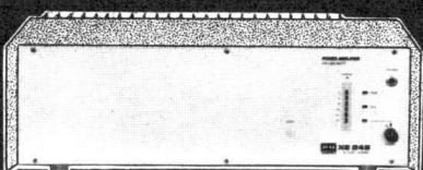
XE 248 Mono-Endverstärker, Netz/Batterie, 320 Watt Musikleistung, 240 Watt Sinusleistung, Übertrager für 4 Ohm, 50/70/100 V eingebaut.
