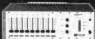
XM 125 Mono-Mischverstärker, Netz/Batterie, 160 Watt Musikleistung, 120 Watt Sinusleistung, Übertrager für 4 Ohm, 50/70/100 V eingebaut.
