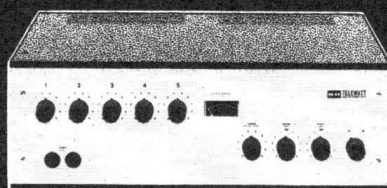
E 120 Mono-Mischverstärker, 160 Watt Musikleistung, 120 Watt Sinusleistung, 100-V-Übertrager nachrüstbar.
