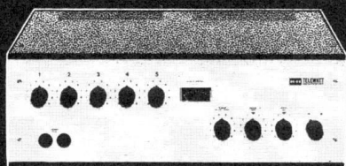
E 60 Mono-Mischverstärker, 80 Watt Musikleistung, 60 Watt Sinusleistung, 100-V-Übertrager nachrüstbar.
