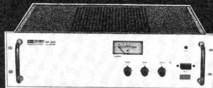
AK 240 Mono-Endverstärker, 320 Watt Musikleistung, 240 Watt Sinusleistung, Über- trager für 4 Ohm, 50/70/100 V eingebaut.
