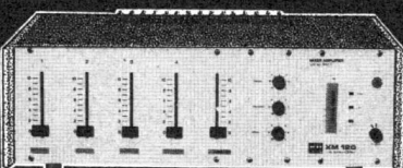
XM 120 Mono-Mischverstärker, Netz/Batterie, 160 Watt Musikleistung, 120 Watt Sinusleistung, Übertrager für 4 Ohm, 50/70/100 V eingebaut.
