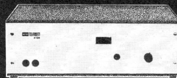
A 120 Mono-Endverstärker, 160 Watt Musikleistung, 120 Watt Sinusleistung, 100-V-Übertrager nachrüstbar.
