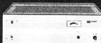
P 120 Mono-Endverstärker, 160 Watt Musikleistung, 120 Watt Sinusleistung, Über- trager für 4/8 Ohm, 50/70/100 V eingebaut.
