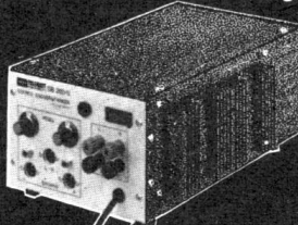
M 126 Mono-Mischverstärker, 160 Watt Musikleistung, 120 Watt Sinusleistung, Über- trager für 4/8 Ohm, 50/70/100 V eingebaut.
