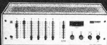
M 126 Mono-Mischverstärker, 160 Watt Musikleistung, 120 Watt Sinusleistung, Über- trager für 4/8 Ohm, 50/70/100 V eingebaut.
