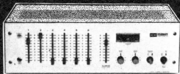
M 66 Mono-Mischverstärker, 80 Watt Musikleistung, 60 Watt Sinusleistung, Über- trager für 4/8 Ohm, 50/70/100 V eingebaut.
