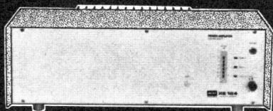
XE 124 Mono-Endverstärker, Netz/Batterie, 160 Watt Musikleistung, 120 Watt Sinus- leistung, Übertrager für 4 Ohm, 50/70/100 V eingebaut.
