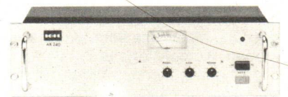
AK 240 Mono-Endverstärker 320 Watt Musikleistung; 240 Watt Sinusleistung 100-V-Übertrager eingebaut
