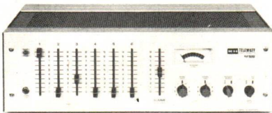
M 66 Mono-Mischverstärker 80 Watt Musikleistung; 60 Watt Sinusleistung 100-V-Übertrager eingebaut
