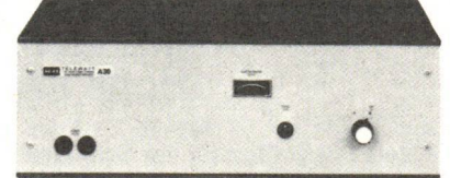
A 120 Mono-Endverstärker 160 Watt Musikleistung; 120 Watt Sinusleistung 100-V-Übertrager nachrüstbar
