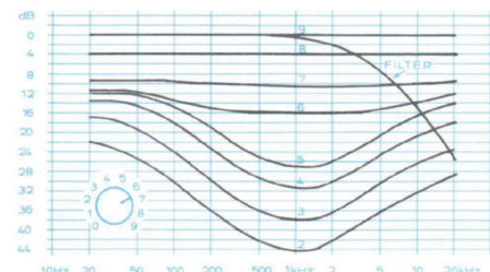
Frequenzgang ES 20 Lautstärkereger (Counter) und Höhenfilter
