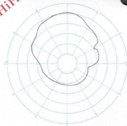
Richtcharakteristik OY bei 10 kHz
