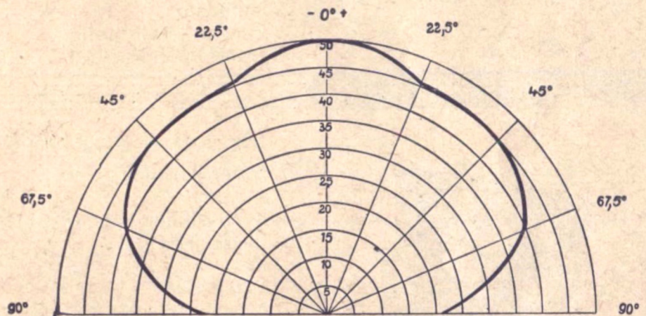
Richtcharakteristik bei 10 000 Hz.
