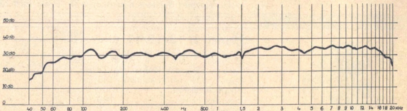
Frequenz-Verlauf der Hoch-Tiefton-Kombination „Orchester“
