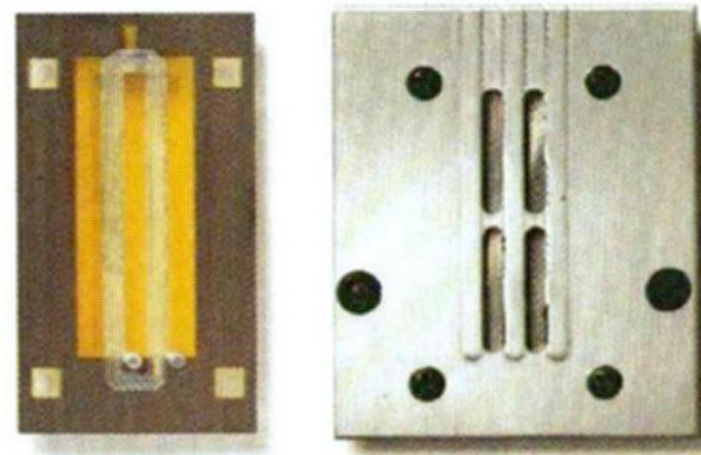
A l'intérieur de notre EMIT un conducteur gravé sur un diaphragme de masse très légère (à gauche) est soumis à deux puissants aimants composés du matériau très rare qu'est le Samarium Cobalt (à droite). Ce nouveau et exclusif HP d'aigu est une amélioration significative en ce qui concerne les performances caractéristiques des conducteurs électrostatiques.
