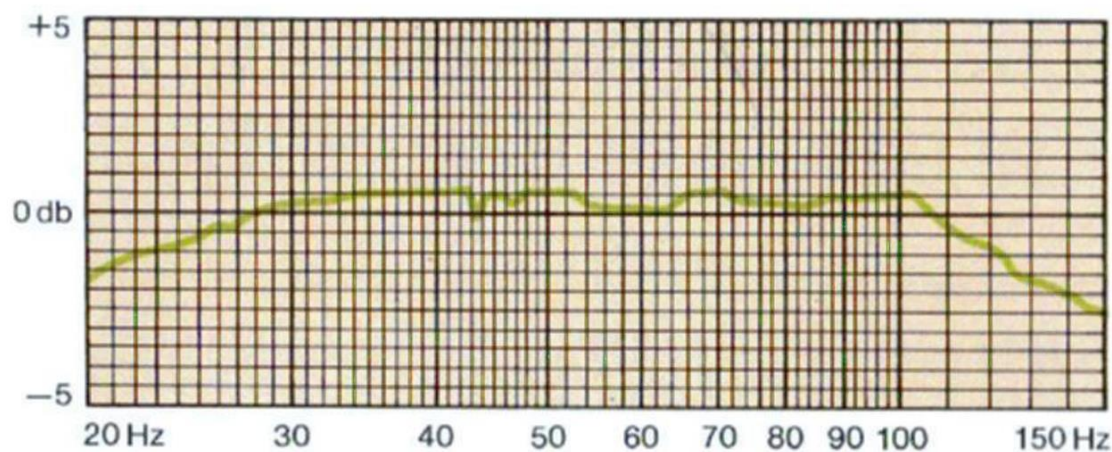
Courbe de réponse des fréquences du HP de basse de la QLS 1, mesurée près du champ et incorporant les pertes de microphone. Courbe de pondération aux environs de 100 Hz, due au filtre.
