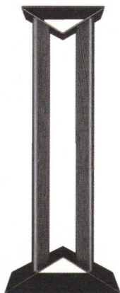
Boxenfuß LS 1 Maße in cm Höhe 63,0 Breite x Tiefe oben 18,0 x 23,0 Breite x Tiefe unten 25,0 x 25,8 Unverb. Preisempfehlung Paar: DM 500,- (Ausführung Eiche schwarz)
