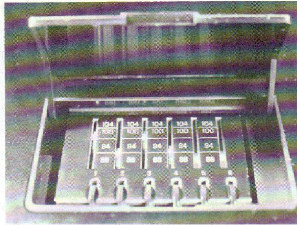
Dissimulés par une trappe située sur le dessus de l'appareil, les six « mini cadrans » de pré réglage des stations M.F.
