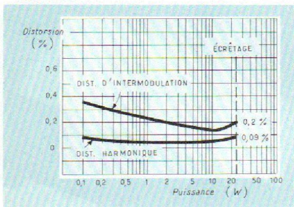
Taux de distorsion harmonique et d'intermodulation.
