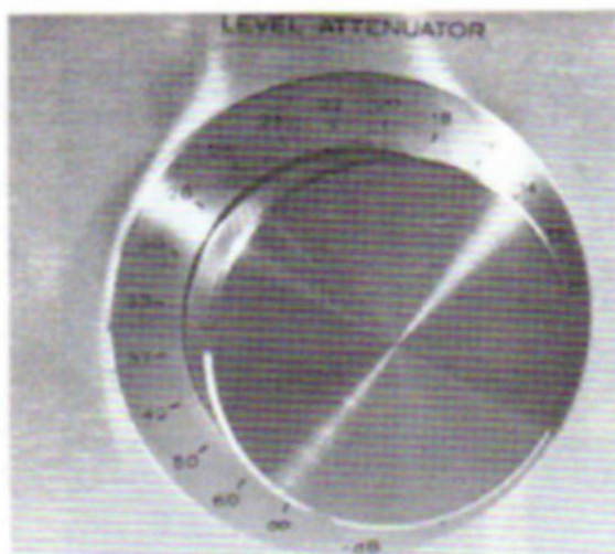
Le réglage du gain est effectué par un gros contacteur à plots.
