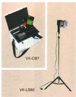
VK-CB7 Schaumstoff-gepolsterter Metallkoffer für Videovieie, Kamera und Zubehör. Abmessungen (BxHxT): 430x325x300 mm.
