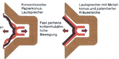
Lautsprechervergleich Papierkonus: Metallkonus/Kräuselsicke
