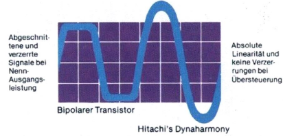
Graphische Darstellung; Simulierte Oszillogramme aus dem Hitachi-Laboratorium in Toyokawa
