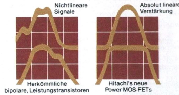
Graphische Darstellung: Simulierte Oszillogramme aus dem Hitachi Laboratorium in Toyokawa
