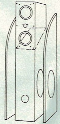
Tief- und Mittel-/Hochtoneinheit arbeiten harmonisch ohne gegenseitige Beeinflussung in zwei getrennten Kammern
