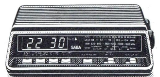
Saba Kompaktclock A , Uhrenradio, UKW/MW, 24-Stunden-Weckautomatik, Nachweckautomatik alle 10 Minuten, Gangreserve bei Stromausfall, verschiedene Farben. 148.-
