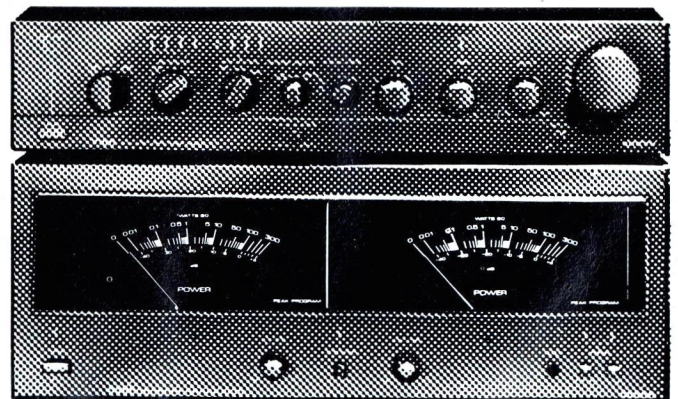
Onkyo P 3060 R Vorverstärker 1300.- Onkyo M 5060 R Endverstärker 2200.- Super-Servo-Regelkreis zur Verbesserung der Raum- und Tiefenstaffelung MM/MC Phono, 3fach Anpassung für MC-System, 2xTB und Copy,
