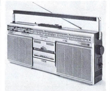
Philips D 8110 , Stereo-Radiorecorder, UKW/MW, Stereo-Weitwinkel, automatische Bandendabschaltung für alle Bandlauffunktionen, Inter-mix-Bedienung, Cue/Review. 2 eingebaute Mikrofone, Teleskopantenne. Netz/Batterie. 248.-
