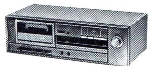
Fisher CR 115, Dolby , Servo-Laufsteuerung über Soft-touch-Tasten, Gleichlaufschwankungen <0,04%, 30-19.000 Hz / Metall. 298.-
