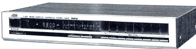
JVC T-X 55 , Digital Quarz Synthesizer, 8 UKW/MW-Stationsspeicher, Test Audio 10/82: „sehr gut“. 898.-
