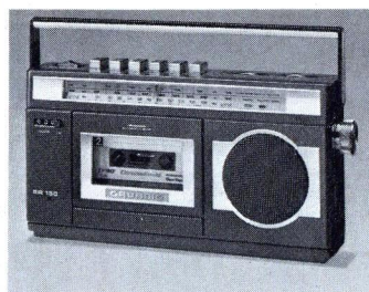
Grundig RR 150 , Radiorecorder, UKW/MW/LW, LED-Anzeige für optimales Tuning, eingebautes Mikrofon, Teleskop- und Ferritantenne. Automatische Bandendabschaltung mit Motorstop und Tastenauslösung. Cue/Review, rastbarer schneller Vor- und Rücklauf. Netz/Batterie. 228.-
