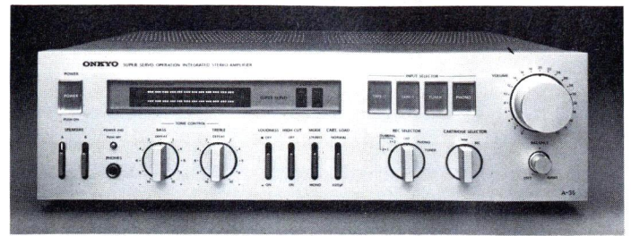
Onkyo A 35, Super-Servo- Vollverstärker, 2 x 90 Watt Sinus, Übertragungsbereich 2 Hz—50 kHz \pm 1 dB, Phono MM/MC, 2 x Tape Rec. Selector, 2 Paar Lautsprecher, LED-Spitzenwertmesser. 698.-
