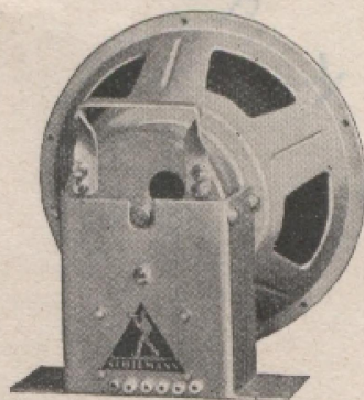
Permanent-dynamische Großlautsprecher-Chassis
