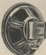
Chassis Perkeo P mit Spezial-Transformator. Benötigt keine Fremd-Erregung. Bis 3 1/2 Watt belastbar. RM 42.—
