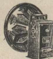
Chassis Cinema mit Ringtauschspule und Spezial- Transformator. Bis 15 W belastbar. Für Gleichstrom | Für Wechselstrom RM 180.— | RM 270.—
