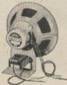
Chassis 10 GI dynamisch für Gleichstrom mit Universal-Anzapfungs- Transformator. RM 26.—
