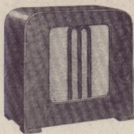
L 58 W, L 58 G Dynamo-Spezial den Mende-Geräten 169, 198, 138 angepaßt. — Bakelite-Gehäuse. RM 58.— Bei Bestellung Apparatstyp und Stromart angeben.
