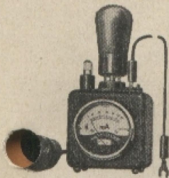
Univ.-Röhren-Prüfgerät
