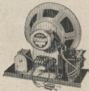
Chassis 10 We dynamisch für Wechselstrom mit Universal-Anzapfungs- Transformator mit Trocken- gleichrichter. RM 48.—
