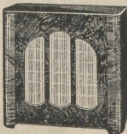
B 16/1 Volldynamischer Lautsprecher mit Universaltrafo für alle Endröhren. Gutes Hartholz-Gehäuse. für Gleichstrom . . . RM 48.— für Wechselstrom, 220 Volt, außerdem notwendig: Hegra- Gleichrichter RG1 . . . RM 7.50 Gleichrichterröhre dazu RM 7.50
