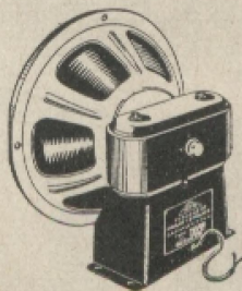
Chassis PMD permanent-dynamisch ohne Fremd-Erregung, mit unterteiltem Transformator. RM 36.—
