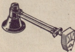
Hegra-Tonabnehmer Mit eingebautem Laut- stärkeregl. Präzisionsarbeit. RM 35.—
